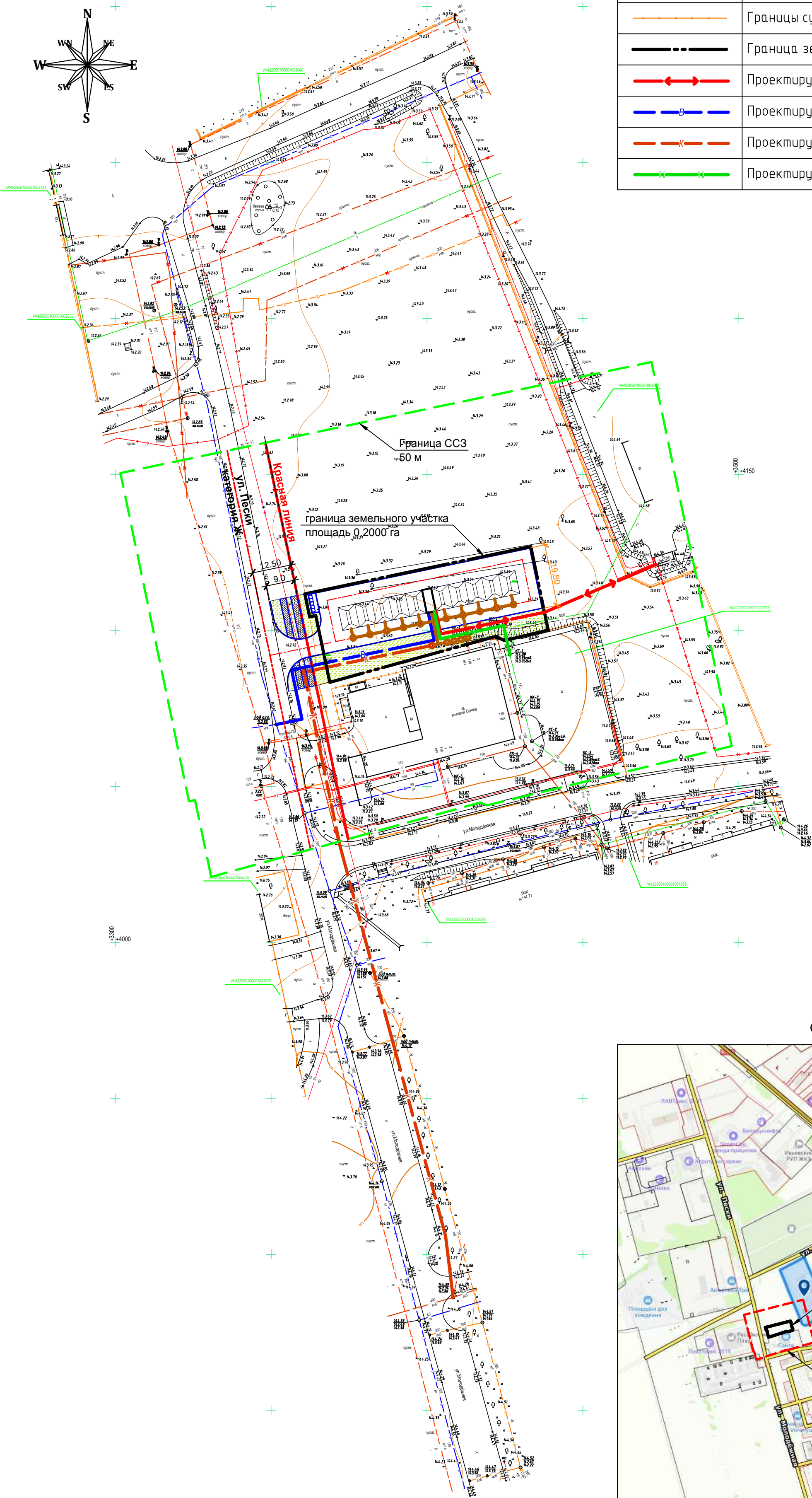
СИТУАЦИОННАЯ СХЕМА
