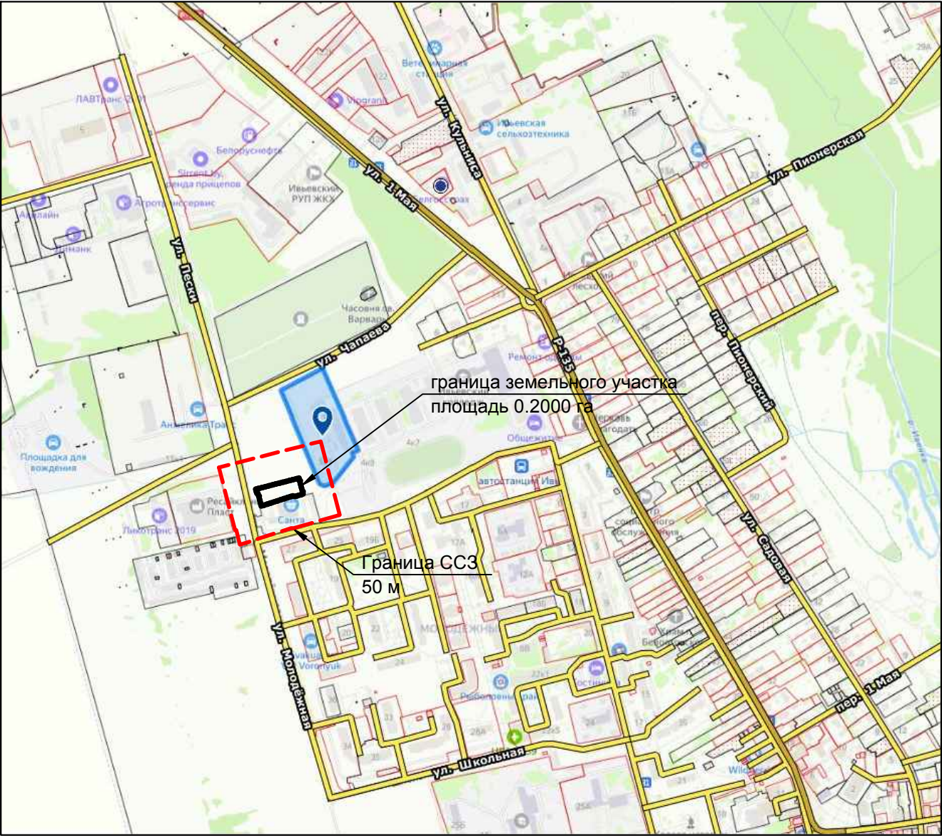
СИТУАЦИОННАЯ СХЕМА
